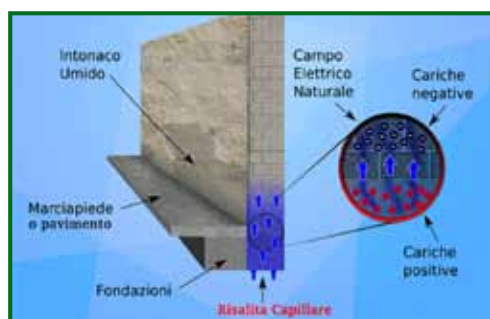
Render spaccato di un muro con presenza di umidità
